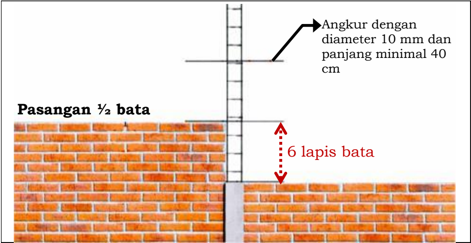
Gambar 46. Hubungan Antara Kolom dengan Dinding
