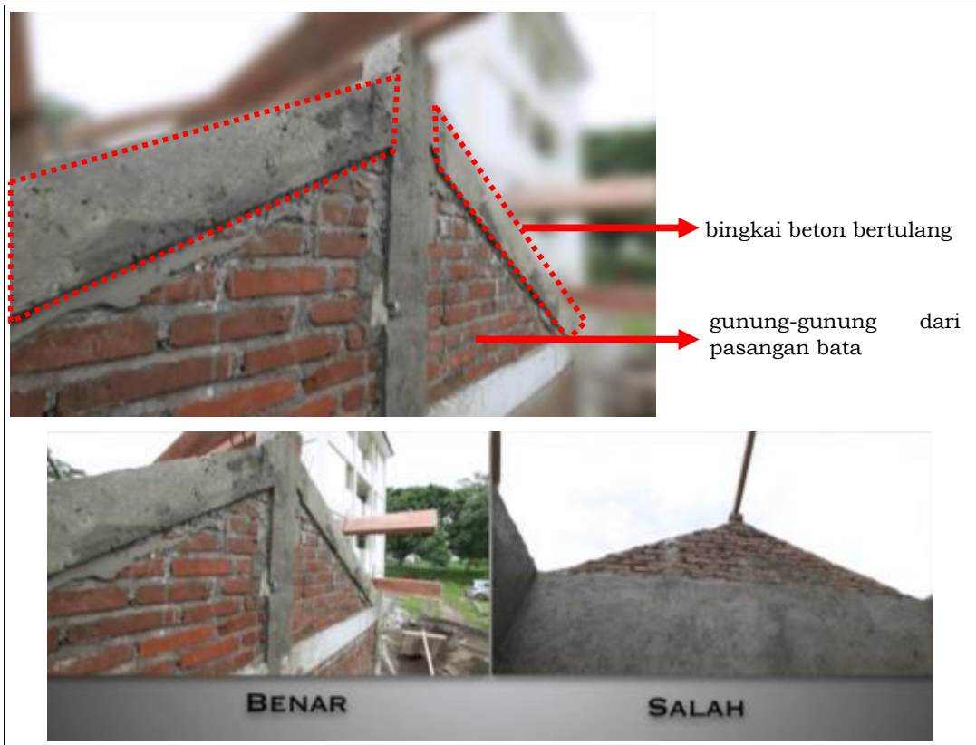
Gambar 32. Gunung-Gunung/ Ampig
