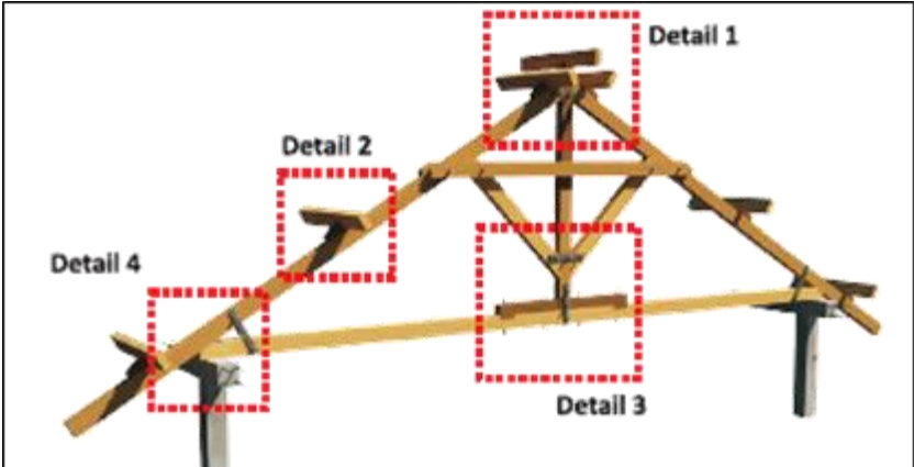
Gambar 25.Kuda-Kuda Kayu
