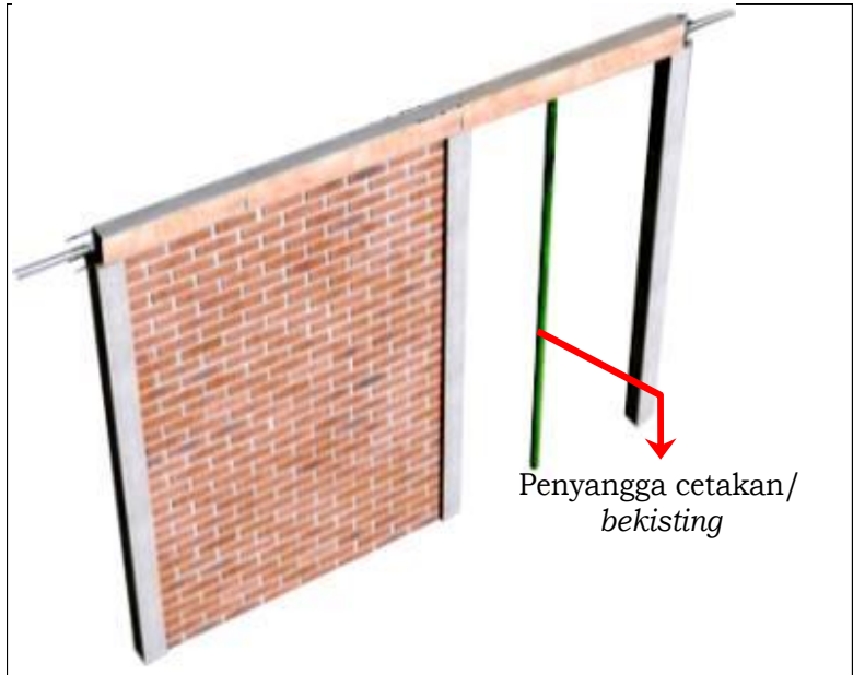
Gambar 60. Penyangga Cetakan/ Bekisting Menggunakan Bambu
